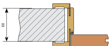
obl. zárubeň B (88-108 mm) síla stěny 90 mm zasunutý záklopový límeček
