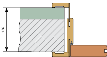
obl. zárubeň B (95-115 mm) síla stěny 126 mm záklopový límeček s delším spojovacím perem +18 mm
