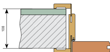
obl. zárubeň B (88-108 mm) síla stěny 110 mm záklopový límeček vysunutý v rozsahu regulace 0-20 mm na své maximum
