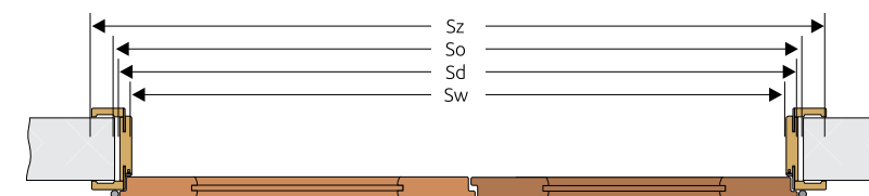
ROZMĚRY REGULOVANÉ ZÁRUBNĚ PRO DVOUKŘÍDLÉ DVEŘE
