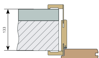
obl. zárubeň B (95-115 mm) síla stěny 133 mm zákloповý límeč s delším spojovacím perem +18 mm
