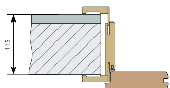
obl. zárubeň B (95-115 mm) síla stěny 115 mm zákloповý límeč vysunutý v rozsahu regulace 0-20 mm na své maximum.
